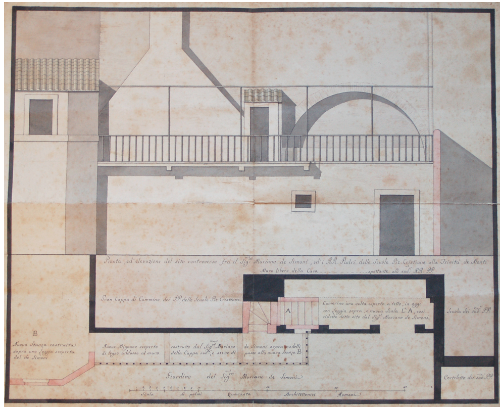
17 Anonymer Aufriß der »Casa dei Preti«. Foto Bibliotheca Hertziana
