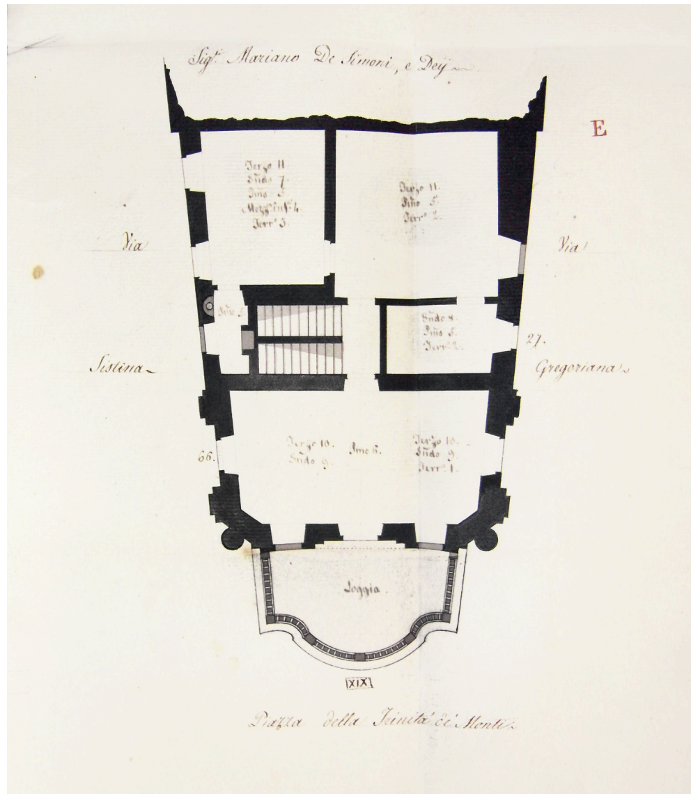
18 Grundriß des ersten Obergeschosses des Tempietto und des Casino. Foto Ministero per i Beni e le Attività Culturali, ASR 23/2013
